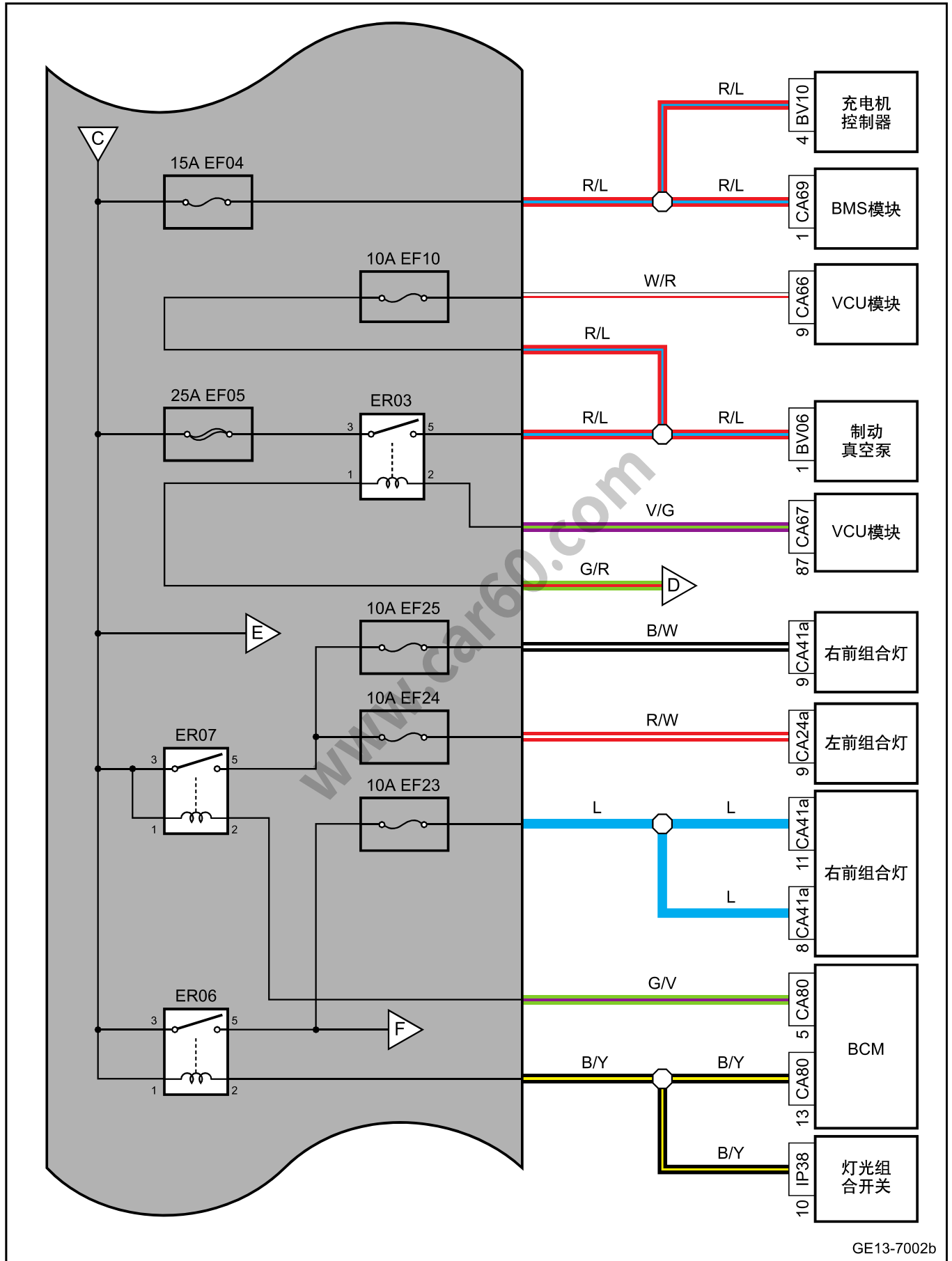
机舱保险丝、继电器盒电源分布图 (续2)
