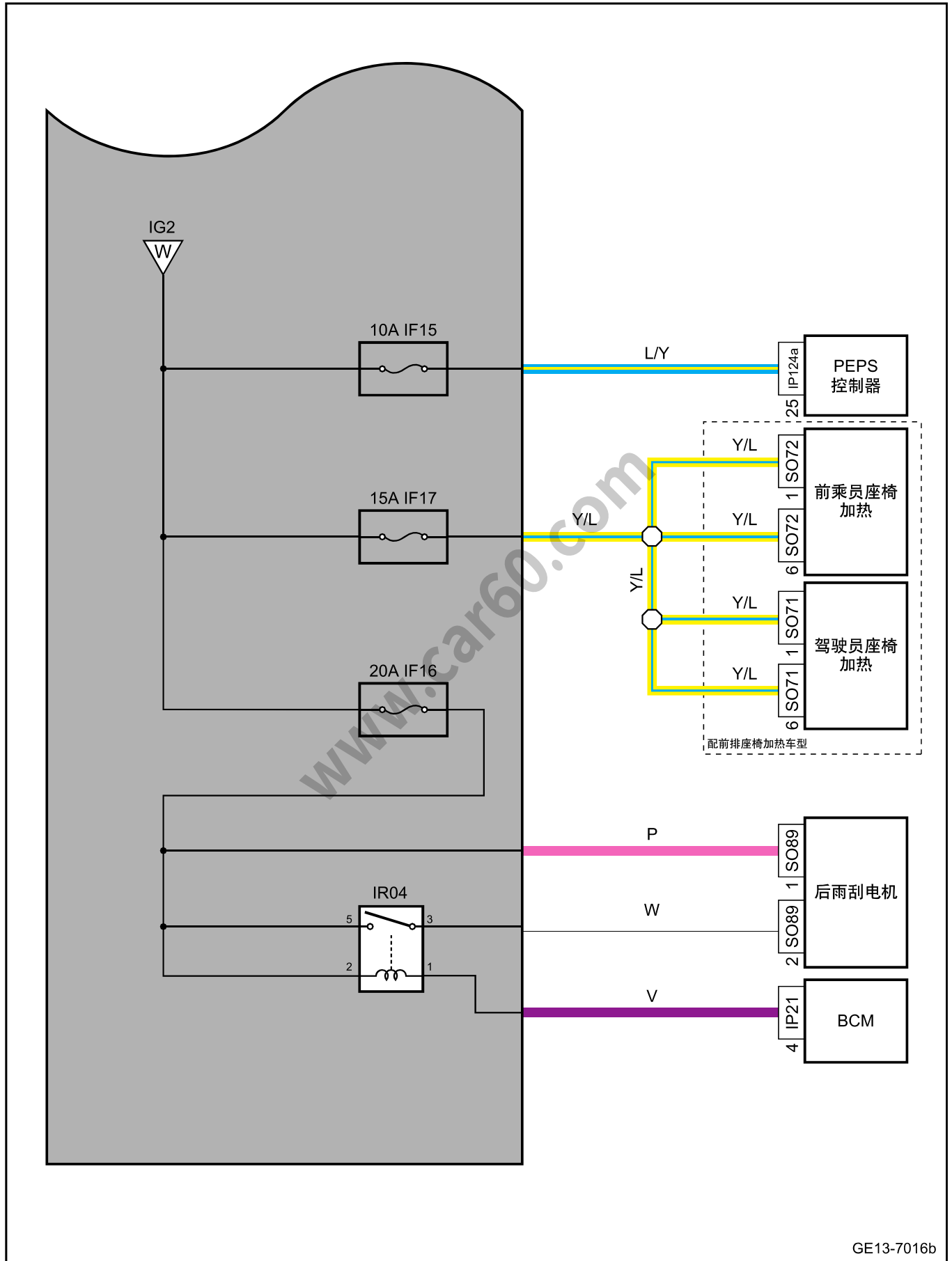
室内保险丝、继电器盒电源分布图（续6）
