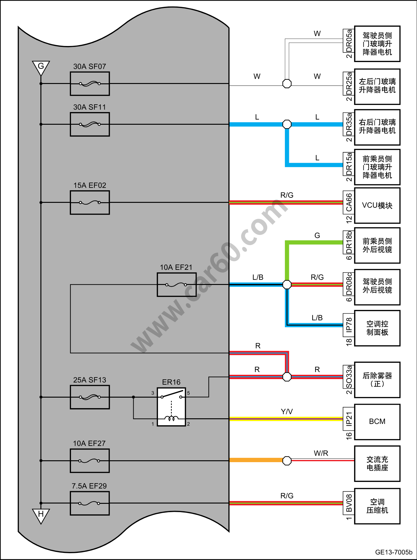
机舱保险丝、继电器盒电源分布图（续5）
