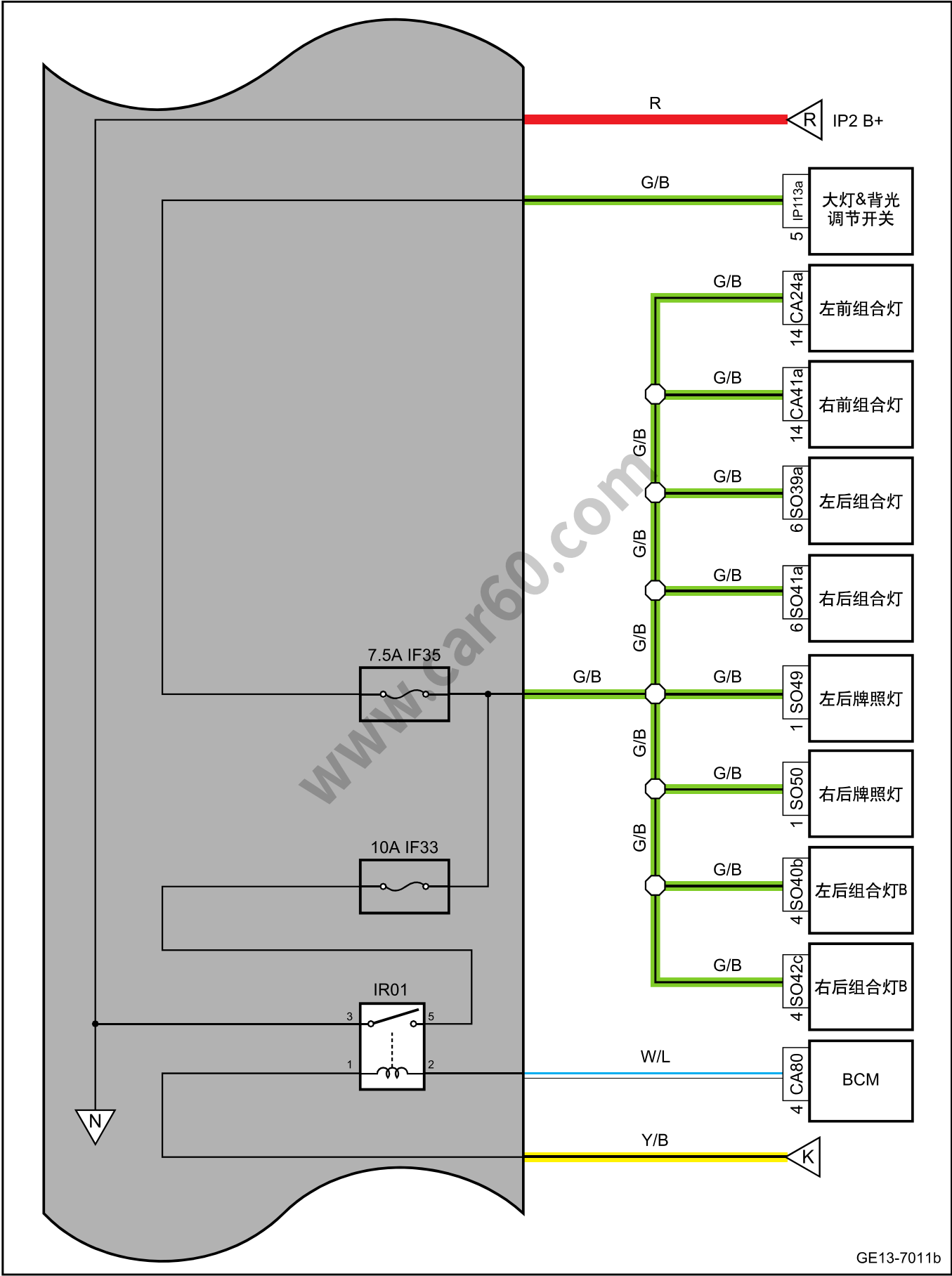
室内保险丝、继电器盒电源分布图(续2 )
