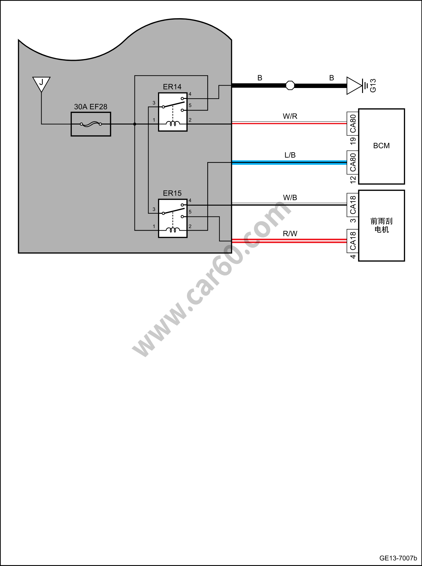
机舱保险丝、继电器盒电源分布图（续7）
