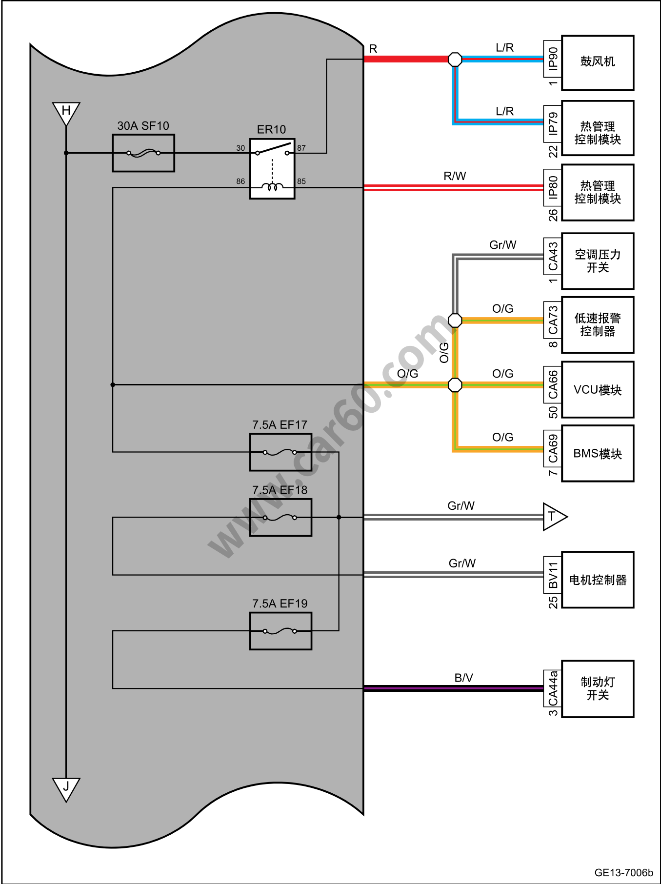
机舱保险丝、继电器盒电源分布图（续6）
