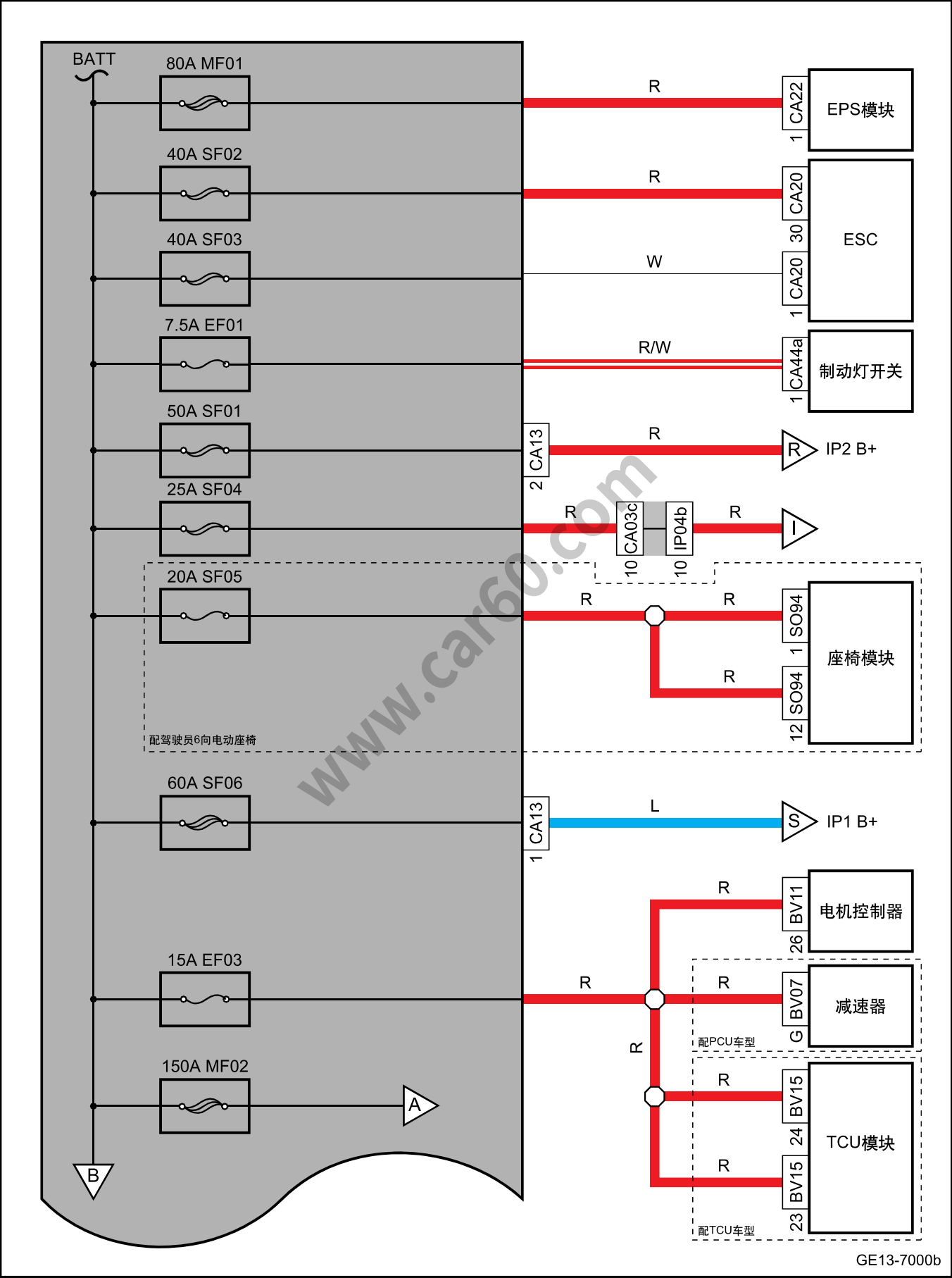
机舱保险丝、继电器盒电源分布图
