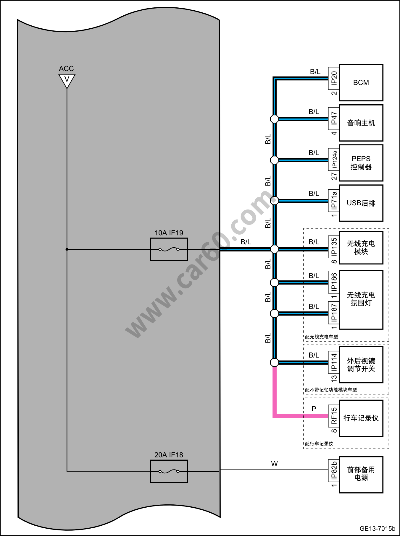
室内保险丝、继电器盒电源分布图（续7）
