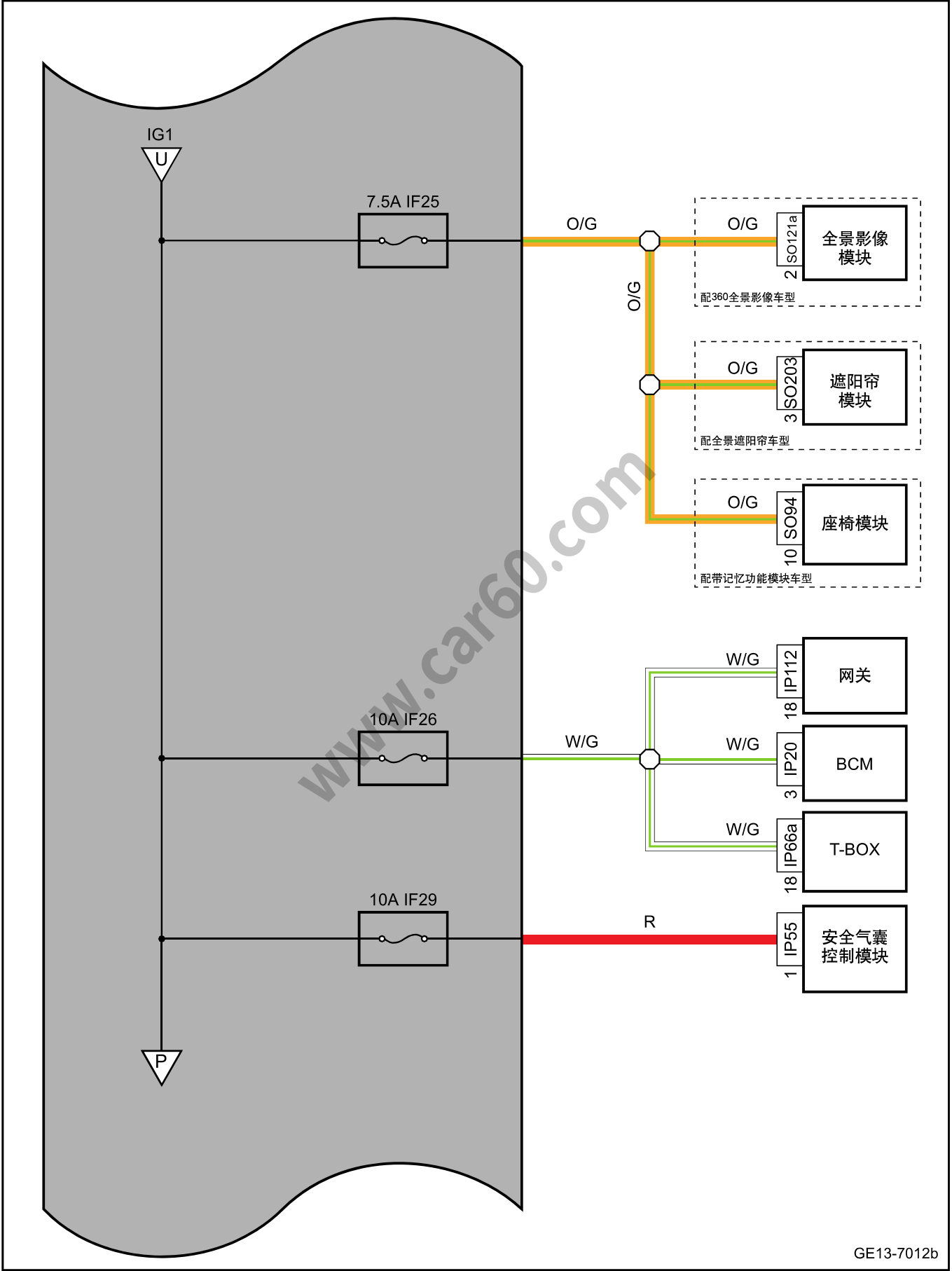
室内保险丝、继电器盒电源分布图（续4）
