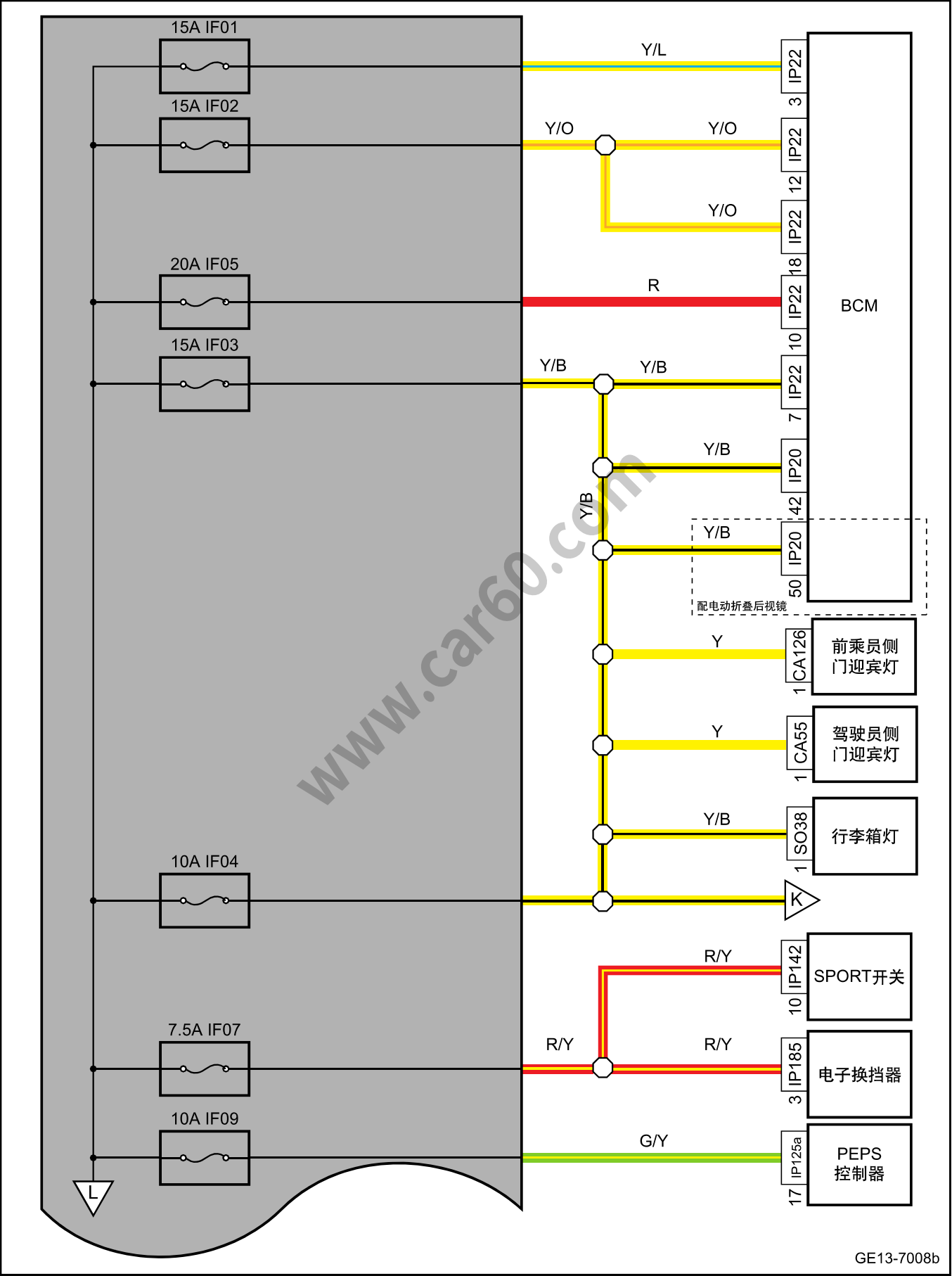
室内保险丝、继电器盒电源分布图
