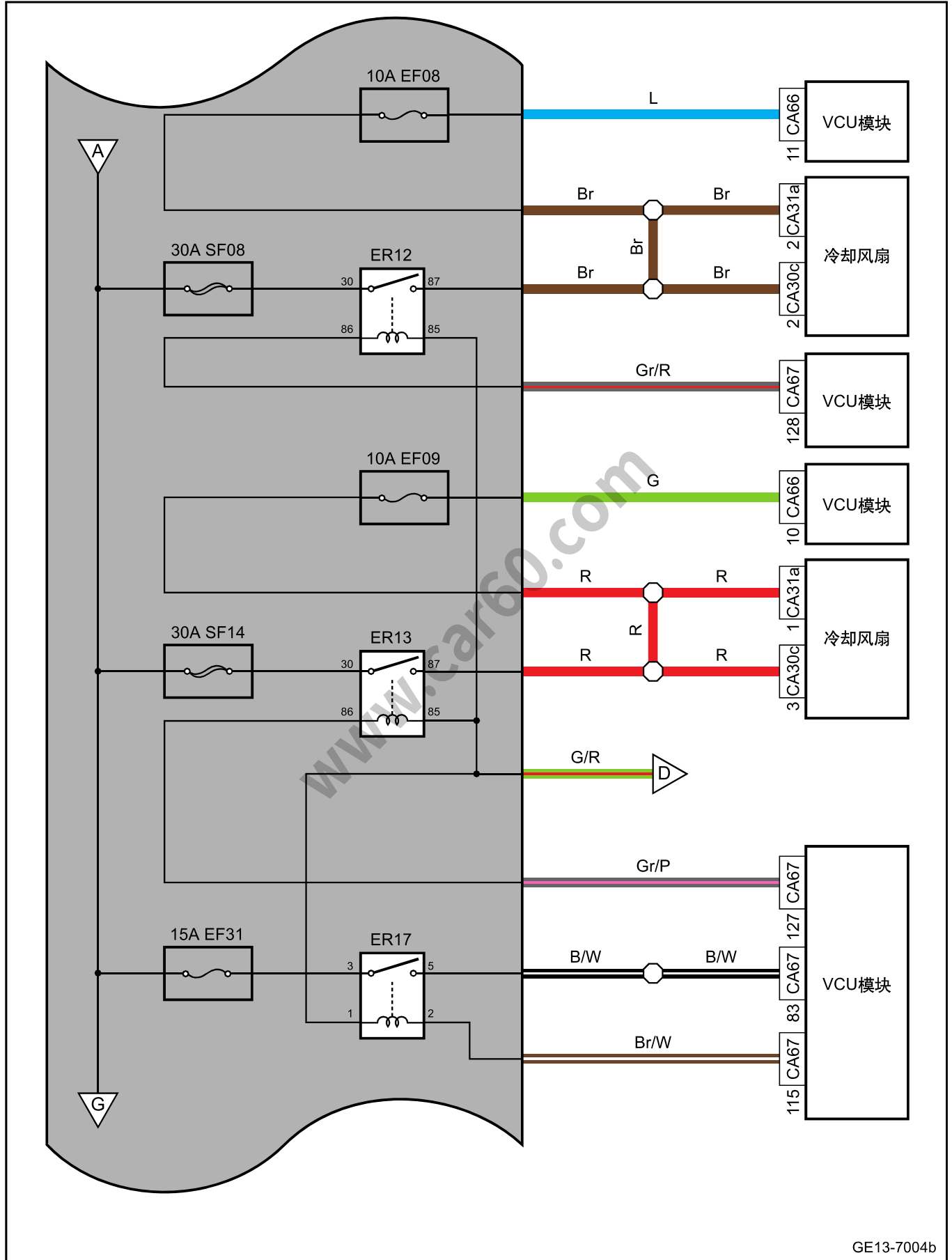
机舱保险丝、继电器盒电源分布图（续4）
