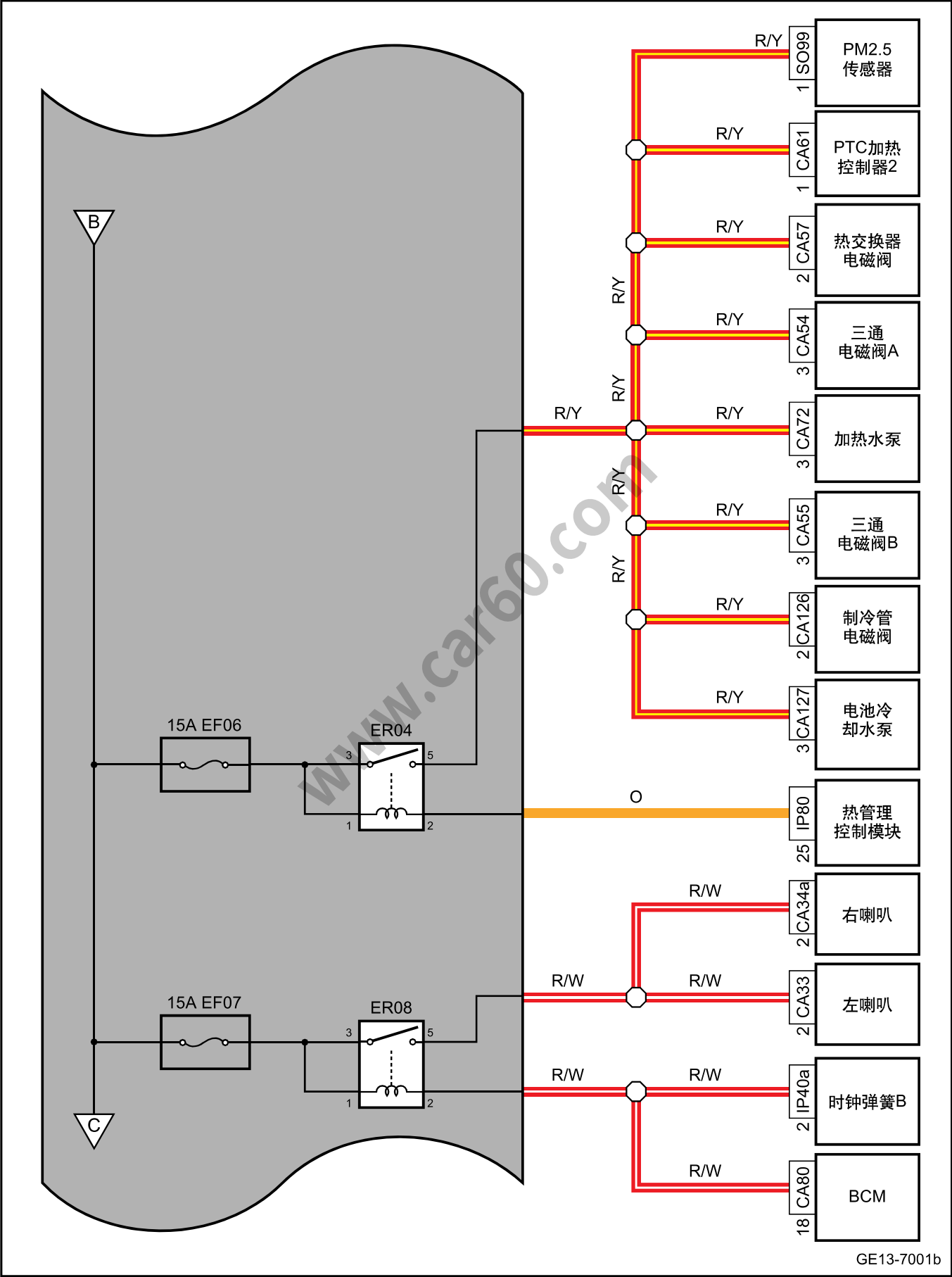
机舱保险丝、继电器盒电源分布图（续1）
