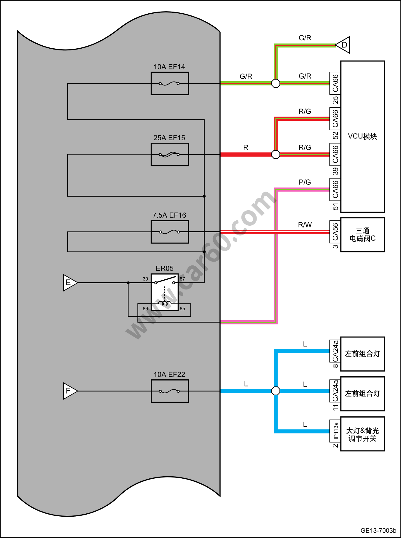
机舱保险丝、继电器盒电源分布图（续3）
